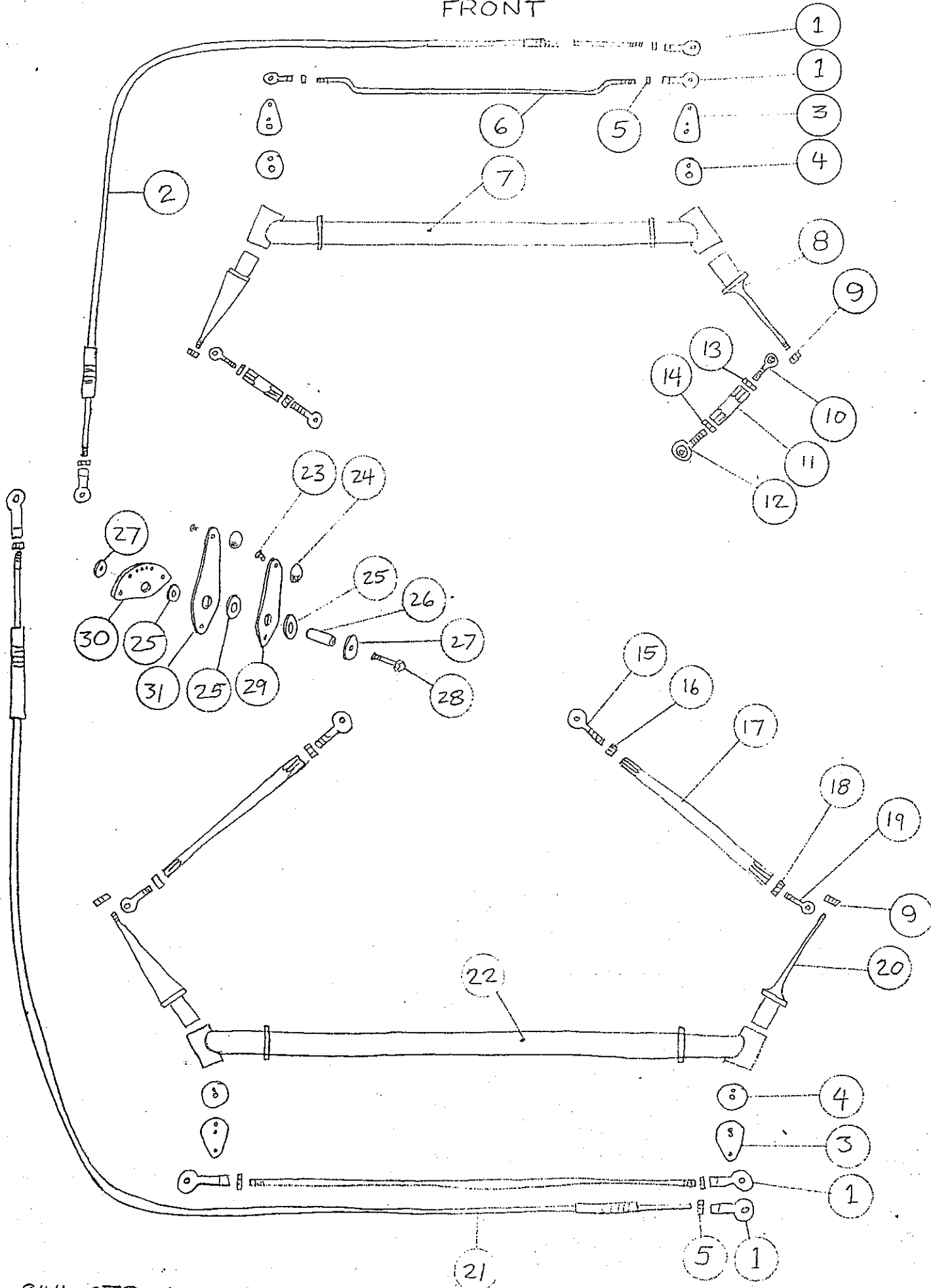
944 GTR ANTI ROLL BAR
